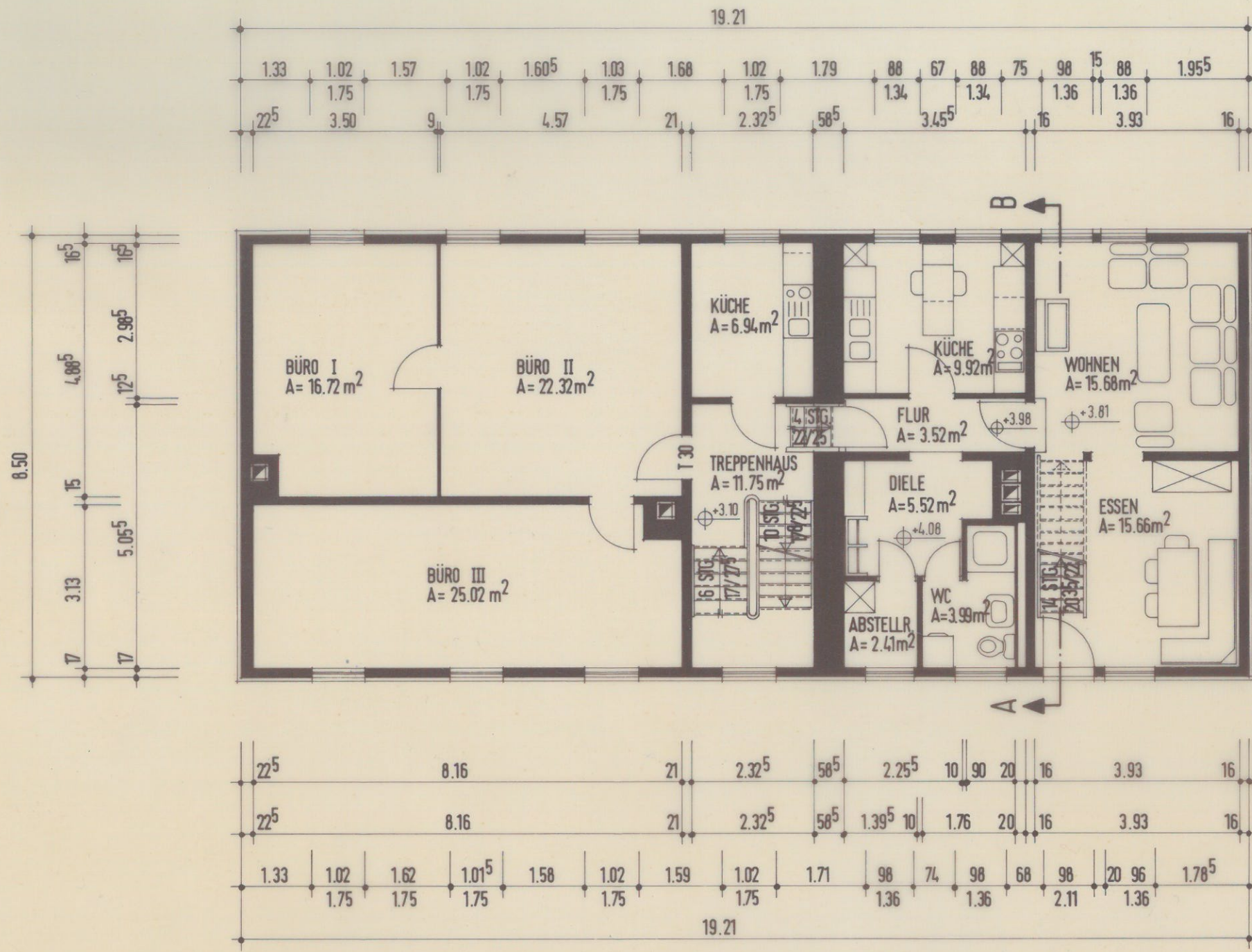
GRUNDRISS 1. OBERGESCHOSS
